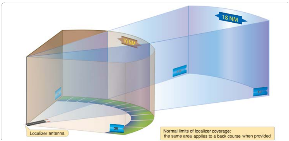
[그림 2-31] Localizer Coverage
