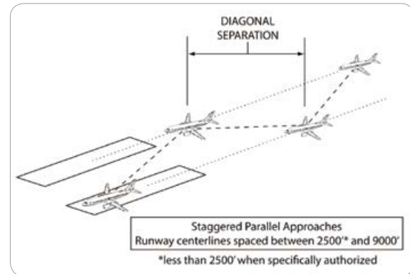
[그림 5-14] Staggered ILS Approaches
