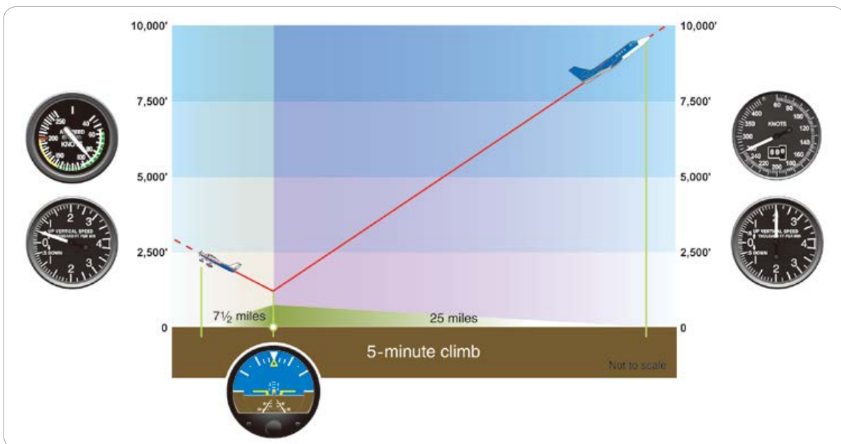
[그림 3-42] Power and altitude equal performance
