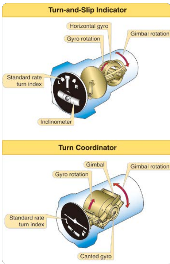
[그림 3-31] turn-and-slip indicator와 turn coordinator
