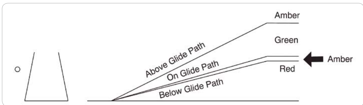
[그림 1-8] Tri-Color Visual Approach Slope Indicator
