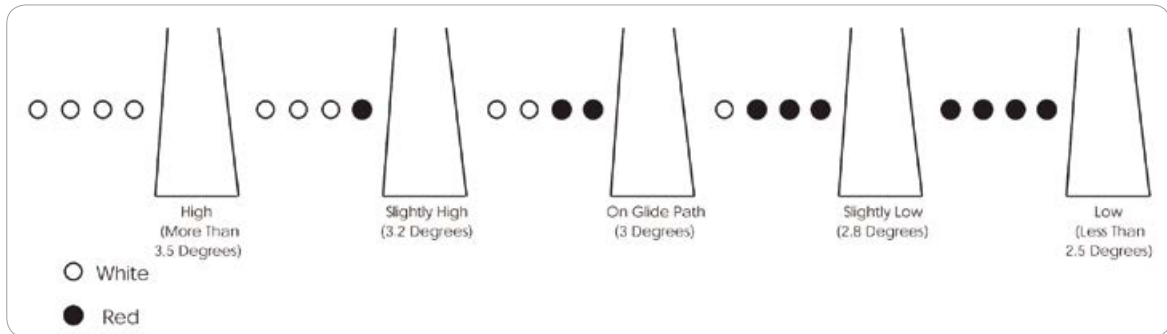
[그림 1-7] Precision Approach Path Indicator (PAPI)
