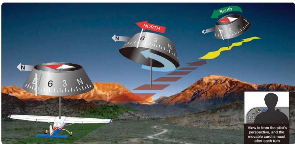
[그림 3-22] 가감속 오차(acceleration error)
