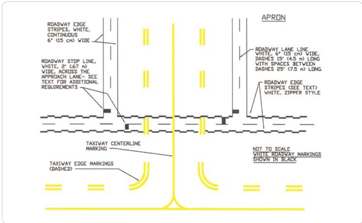
[그림 1-30] Vehicle Roadway Markings
