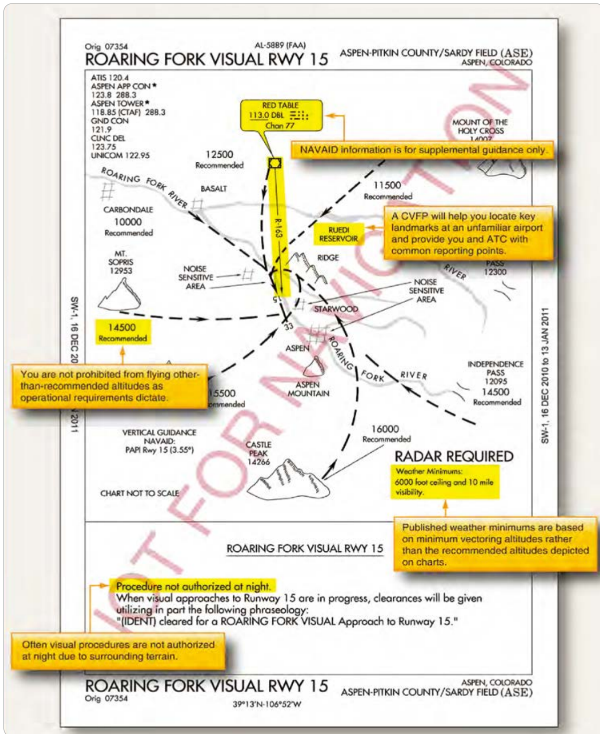
[그림 5-16] Charted visual flight procedures(CVFP)
