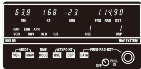
[그림 2-22] Typical RNAV display
