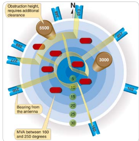
[그림 8-5] Minimum Vectoring Altitude Chart
