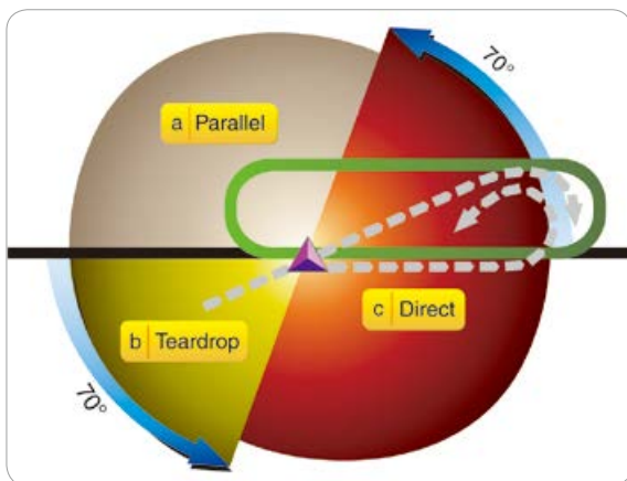
[그림 5-8] Holding Pattern entry procedures
