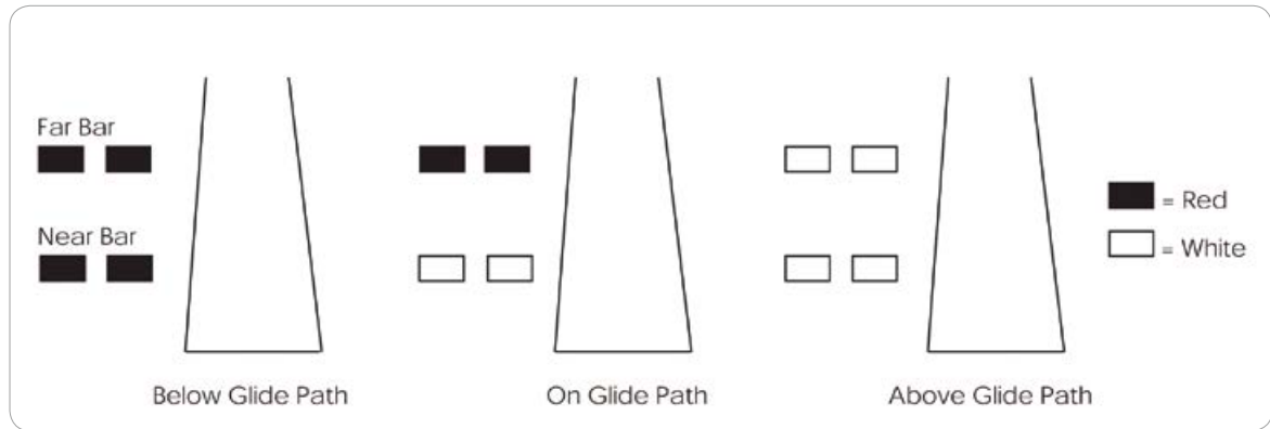
[그림 1-4] 2-Bar VASI
