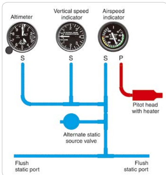
[그림 3-2] A typical pitot-static system
