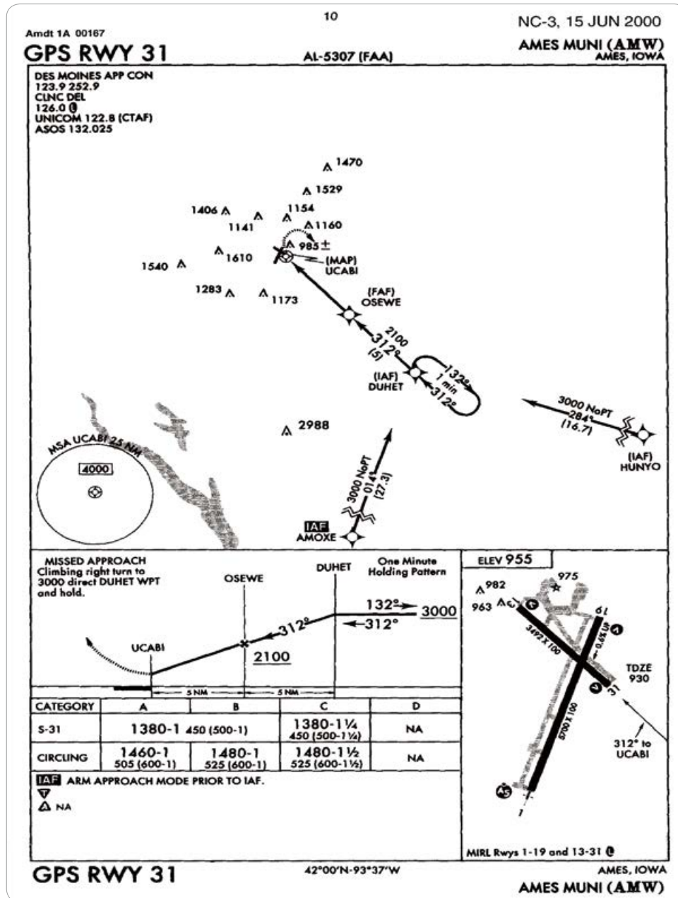
[그림 5-10] Ames, Iowa (AMW) GPS Rwy 31 approach
