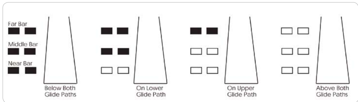
[그림 1-5] 3-Bar VASI
