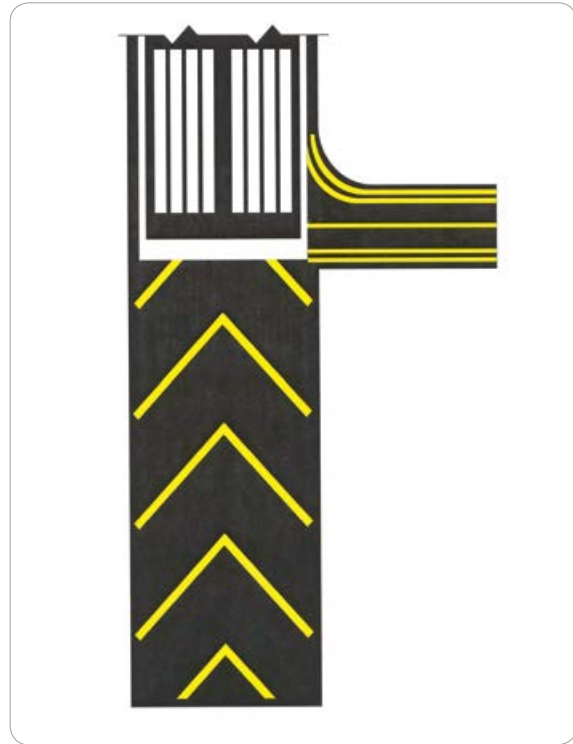
[그림 1-18] Markings for Blast Pads and Stopways
