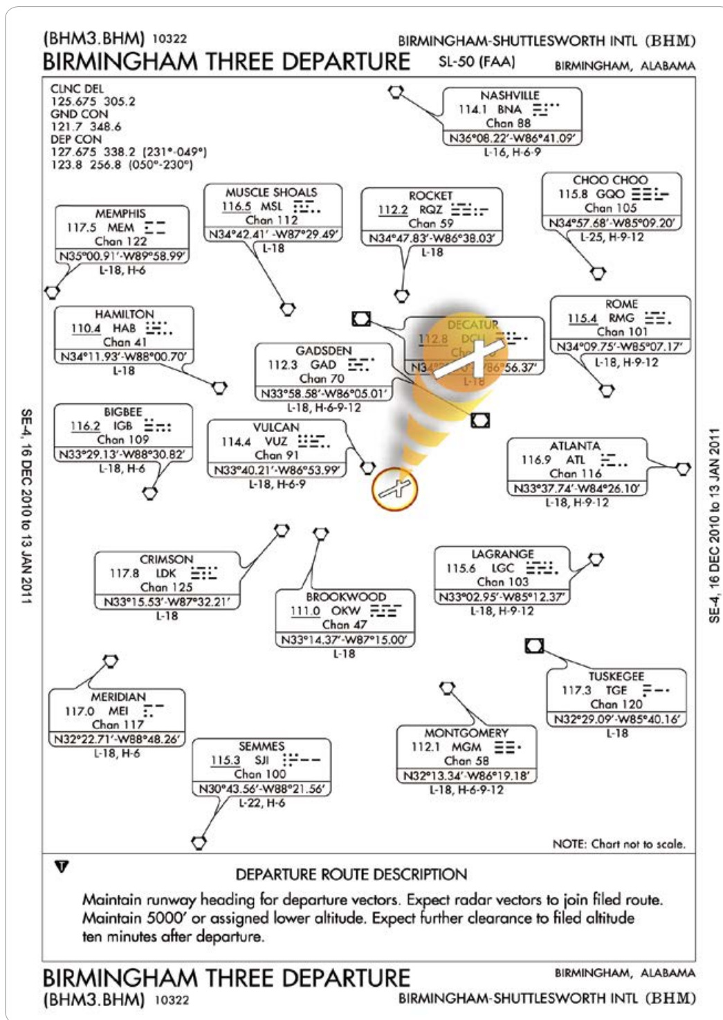
[그림 5-3] Departure Procedure
