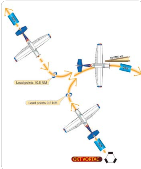
[그림 2-18] DME arc interception
