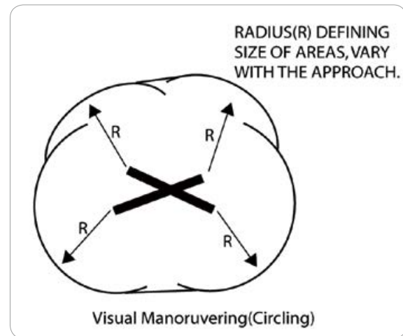
[그림 1-49] 선회 접근구역
