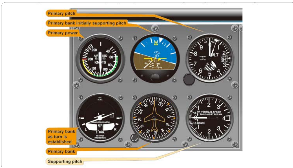
[그림 4-33] Standard-rate turn, constant airspeed
