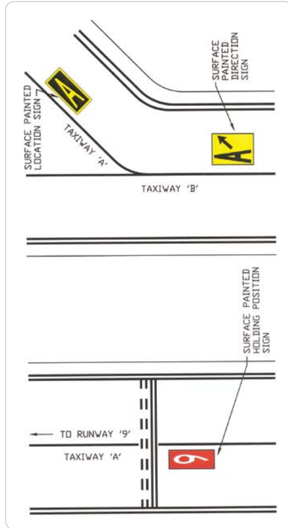
[그림 1-23] Surface Painted Signs
