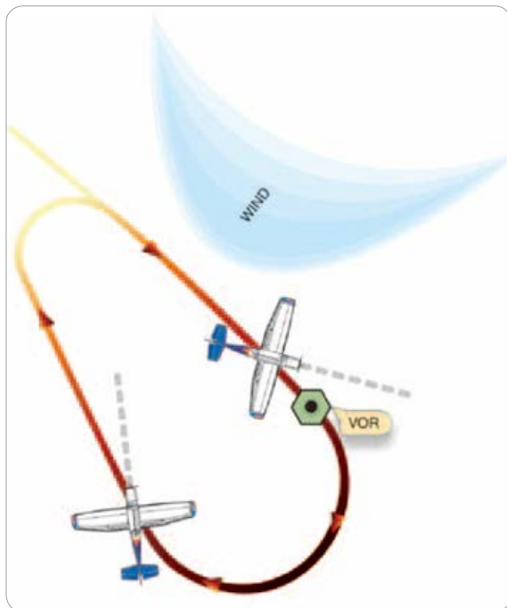
[그림 5-7] Drift correction in holding pattern
