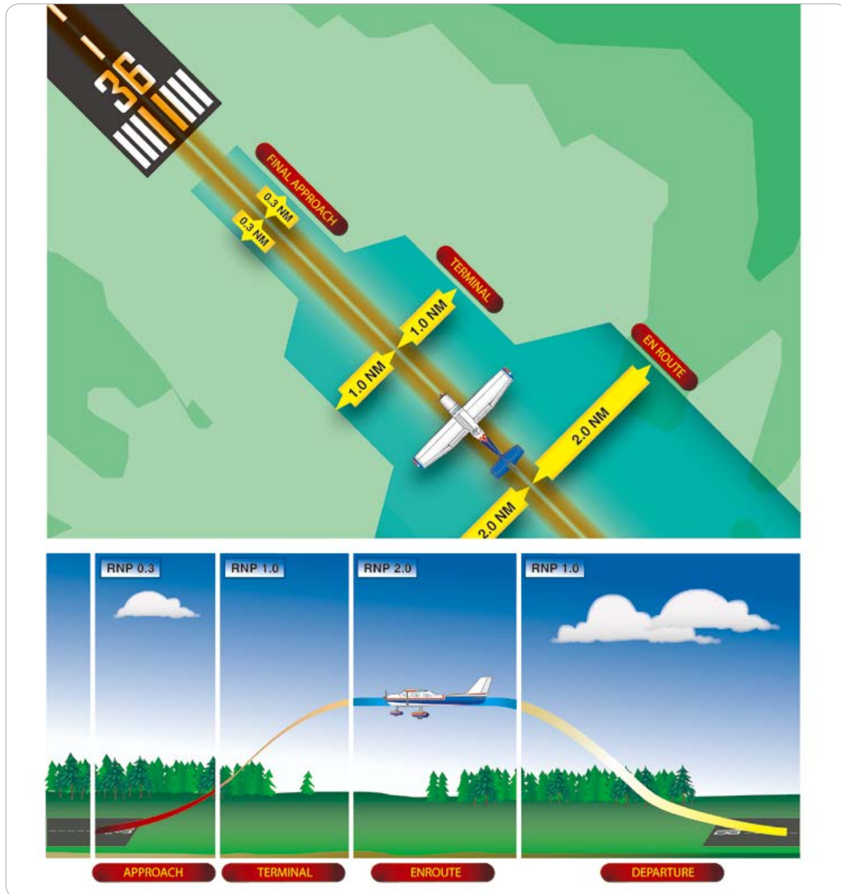
[그림 2-27] Required navigation performance
