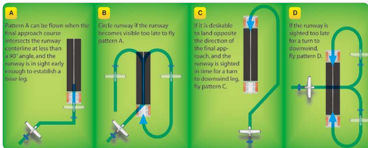
[그림 5-18] Circling approaches
