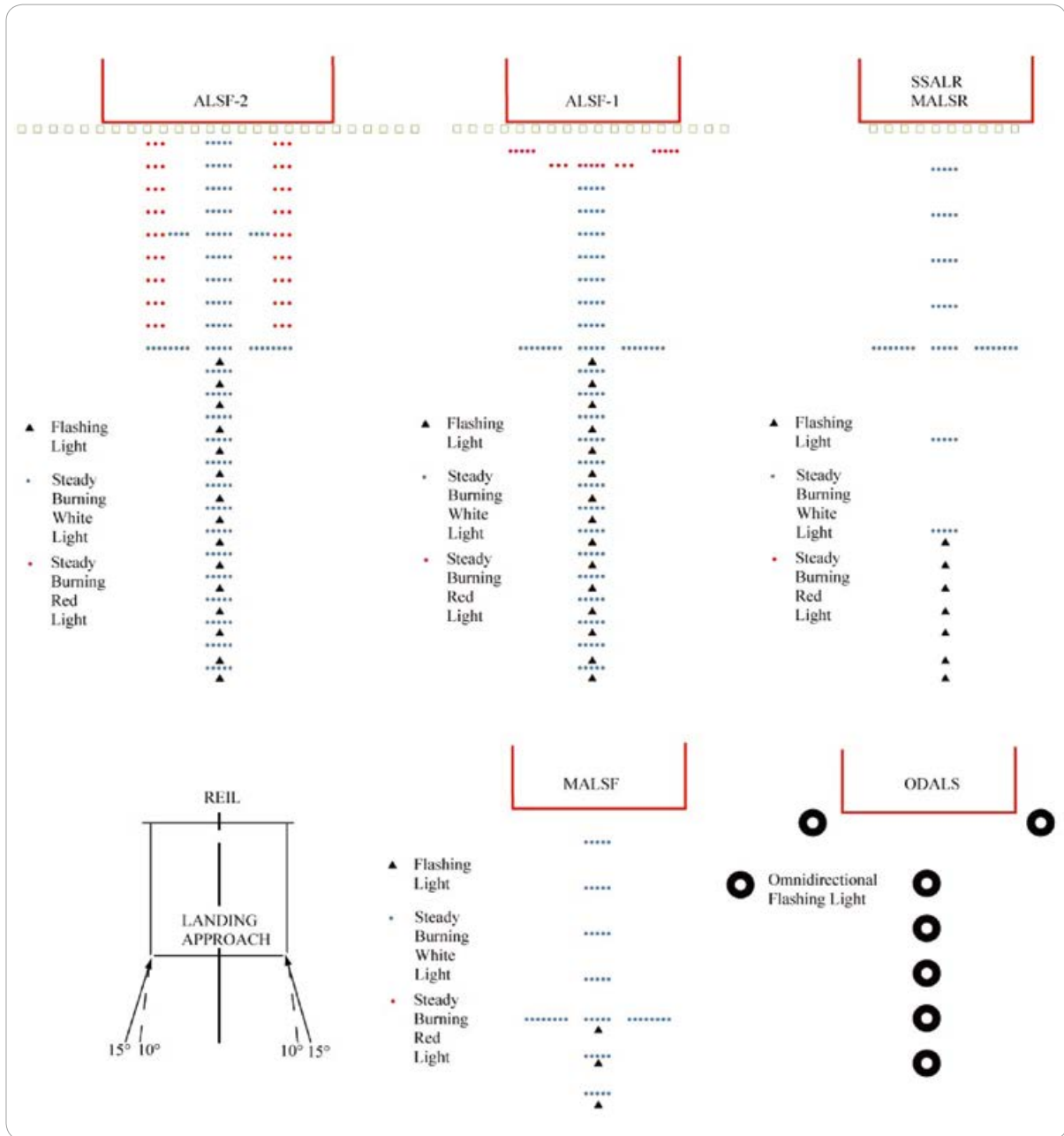
[그림 1-3] Precision & Nonprecision Configurations
