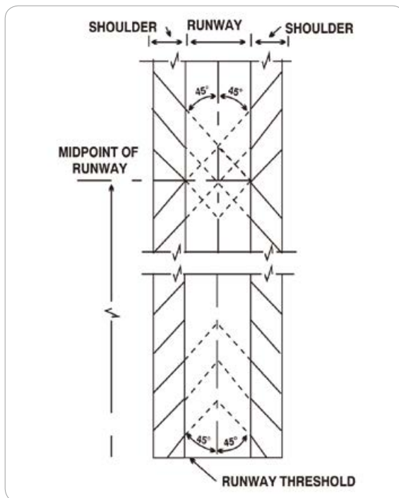
[그림 1-15] Runway Shoulder Markings
