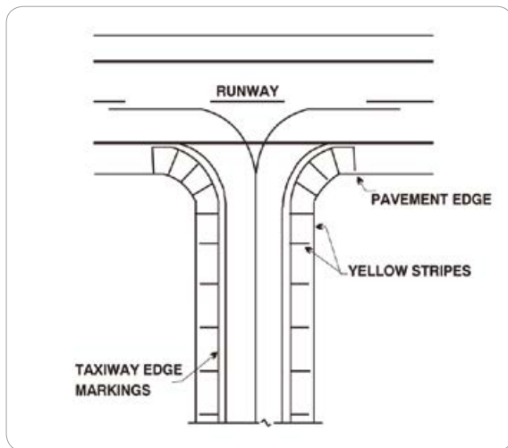
[그림 1-22] Taxi Shoulder Markings
