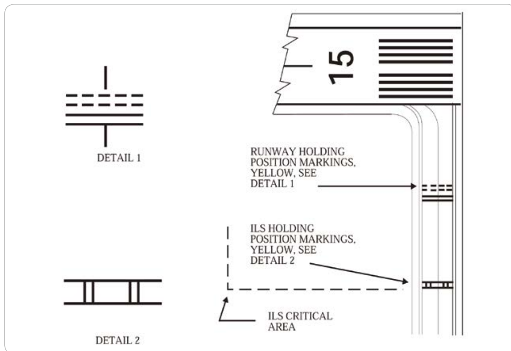
[그림 1-28] Holding Position Markings: ILS Critical Area
