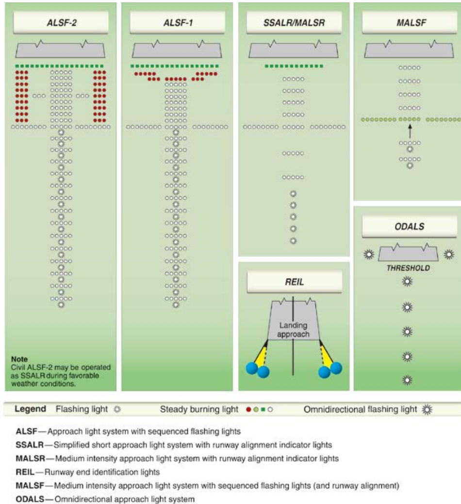
[그림 2-33] Precision and nonprecision ALS configuration
