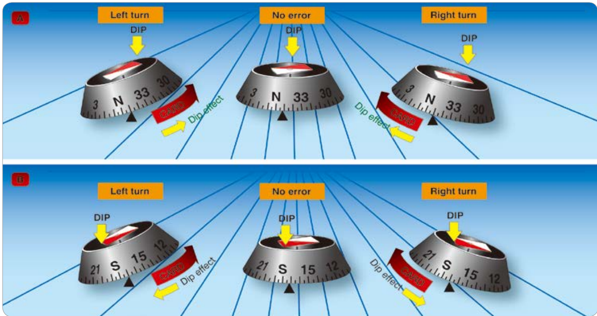
[그림 3-21] 복선 오차(Northerly turning error)
