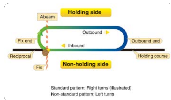
[그림 5-6] Standard holding pattern - no wind
