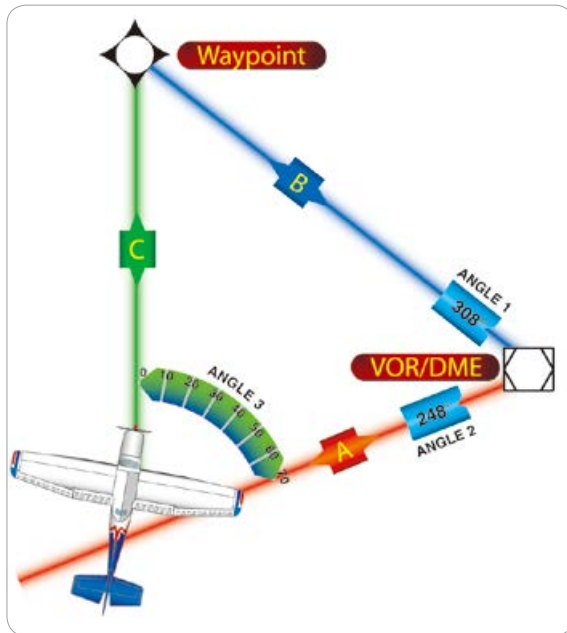
[그림 2-21] RNAV computation
