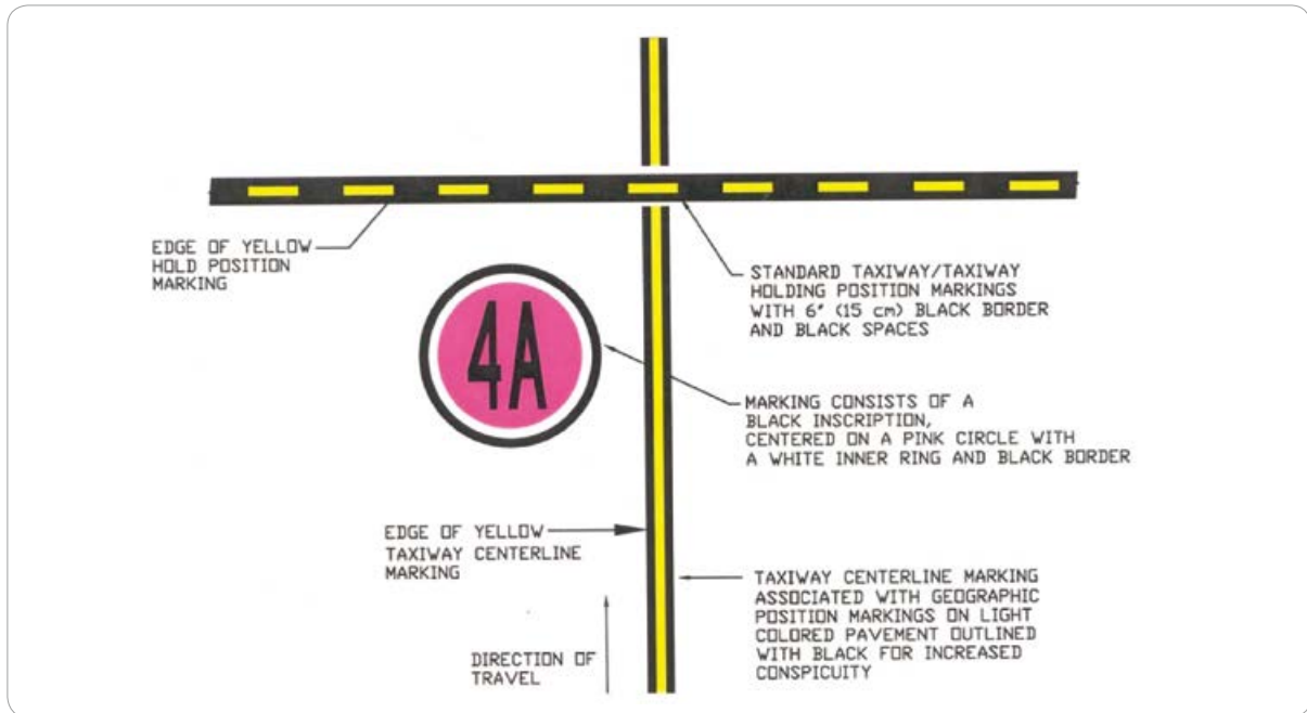
[그림 1-24] Geographic Position Markings
