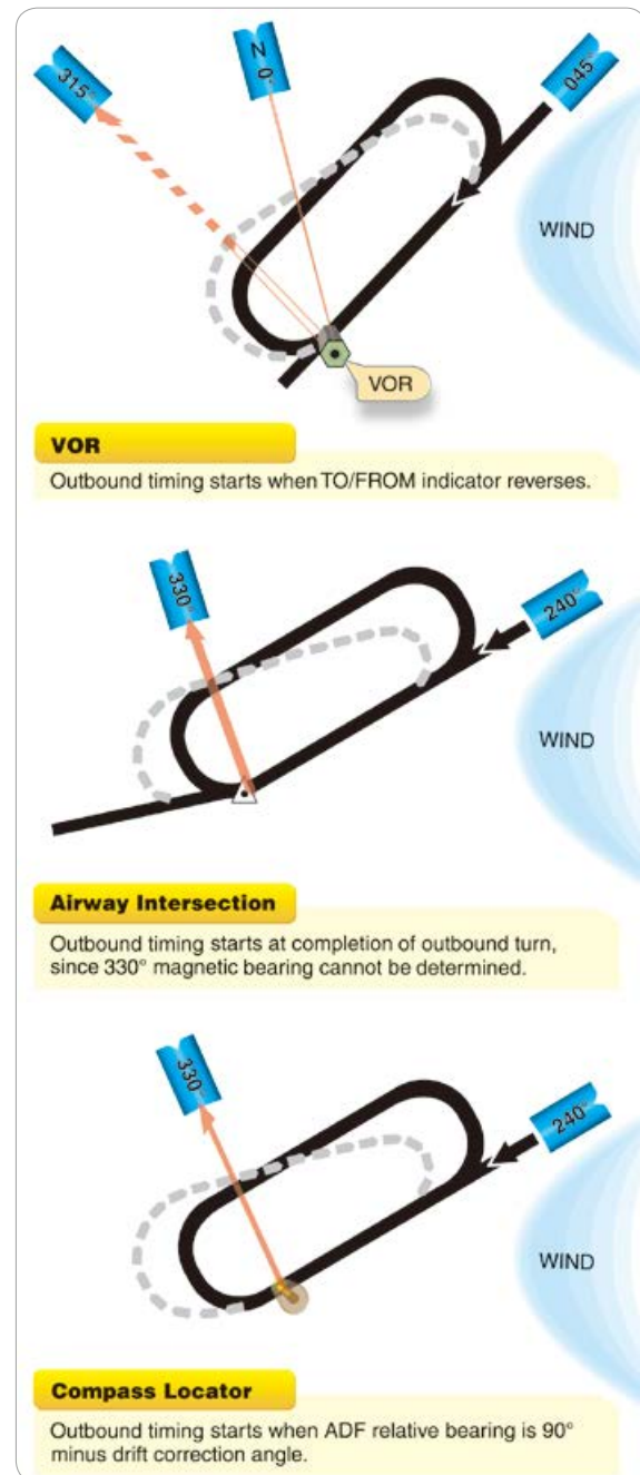
[그림 5-9] Holding - outbound timing
