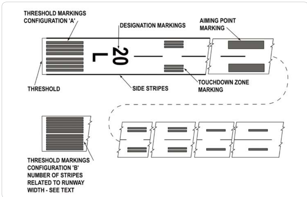
[그림 1-13] Precision Instrument Runway Markings
