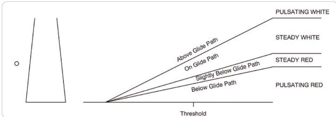
[그림 1-9] Pulsating Visual Approach Slope Indicator
