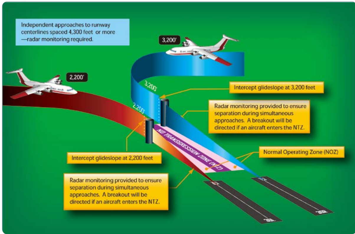
[그림 5-15] Simultaneous Parallel ILS Approaches
