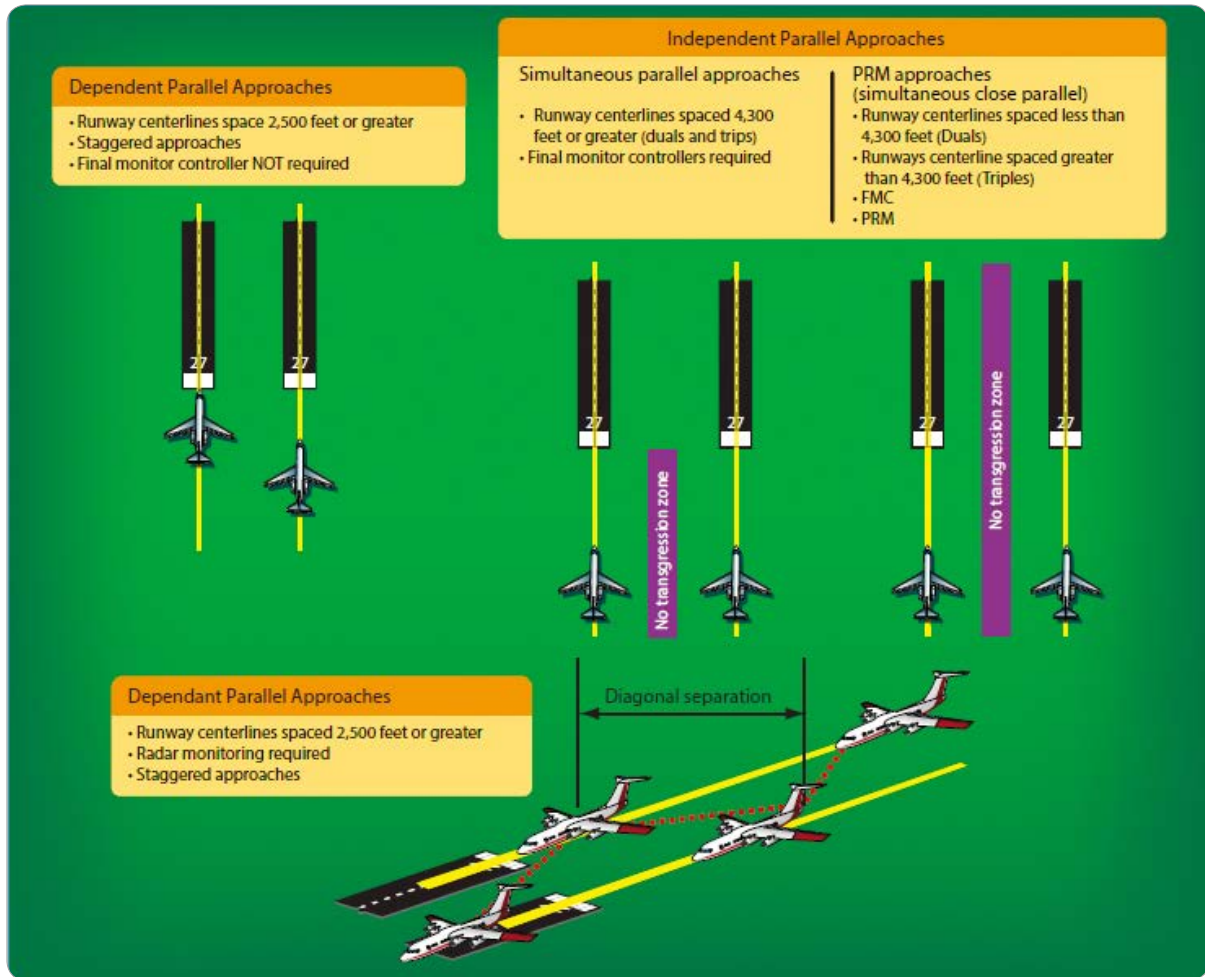
[그림 5-13] Parallel(dependent) ILS approach
