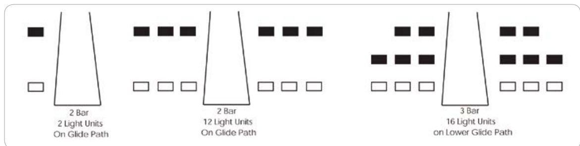
[그림 1-6] VASI Variations
