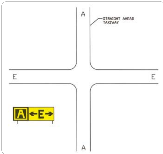
[그림 1-44] Direction Sign Array for Simple Intersection
