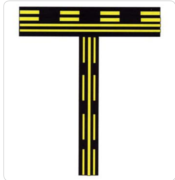
[그림 1-20] Enhanced Taxiway Centerline
